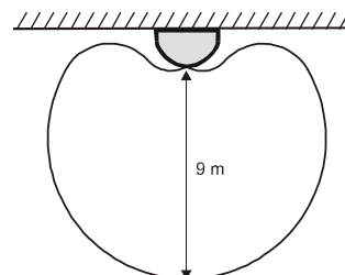
Pole detekcji czujnika zbitcia szkła
