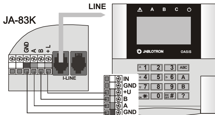
Schemat 1. Podłączenia do centrali alarmowej
