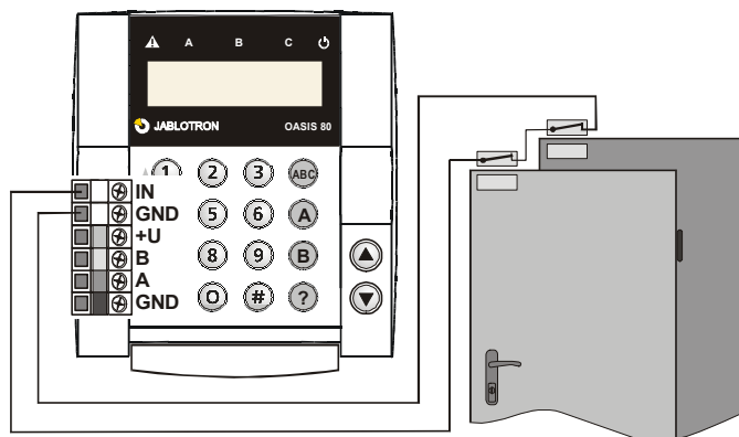
Przykład podłączenia czujnika drzwi
