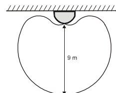
Pole detekcji czujnika zbitcia szkła
