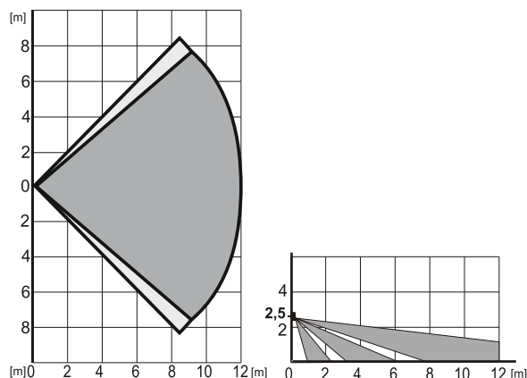
Rys. 2: Charakterystyka detekcji
