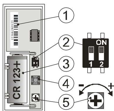
Rysunek nr 3: 1 – numer seryjny; 2 – konfiguracja i tryb pracy; 3 – bateria CR-123A; 4 – styk sabotażowy; 5 – czułość czujnika
