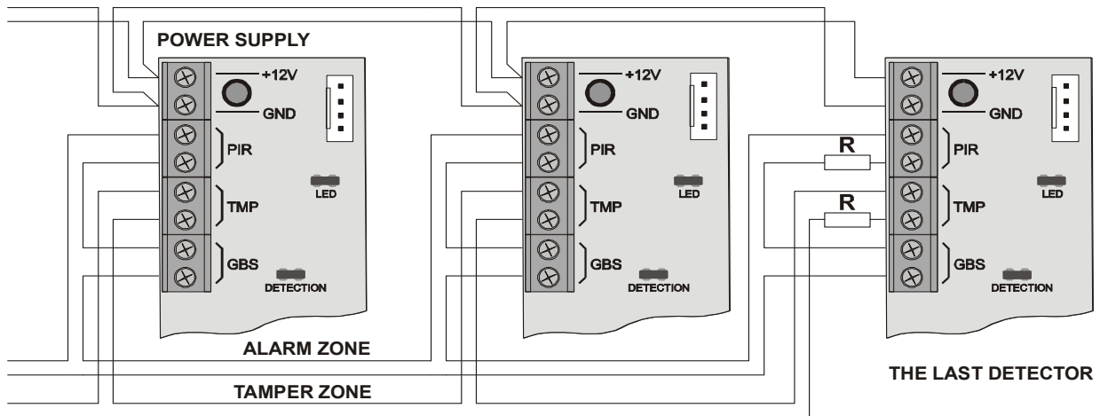
Przykład połączenia kilku czujników na jednej linii w konfiguracji z pojedynczym rezystorem EOL.
