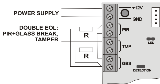
Przykład połączenia czujnika w konfiguracji z podwójnym rezystorem 2EOL
