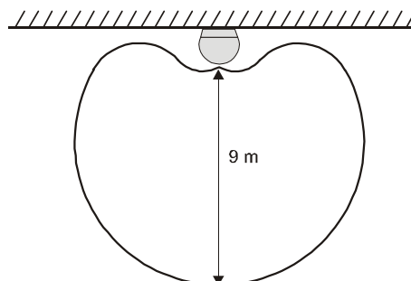
Charakterystyka działania czujnika zbitcia szyby
