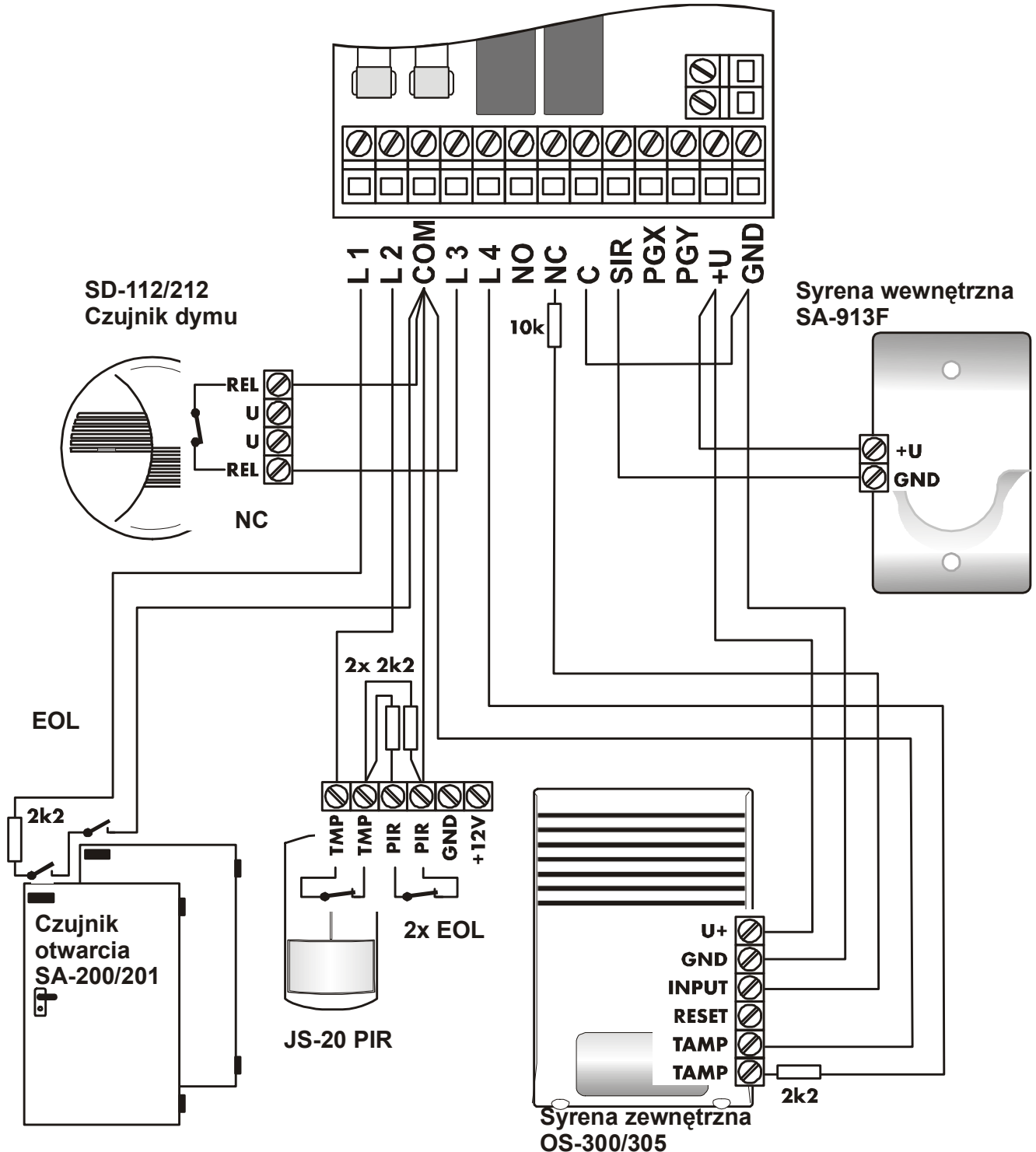
Rys. 1. Połączenia przewodowe
